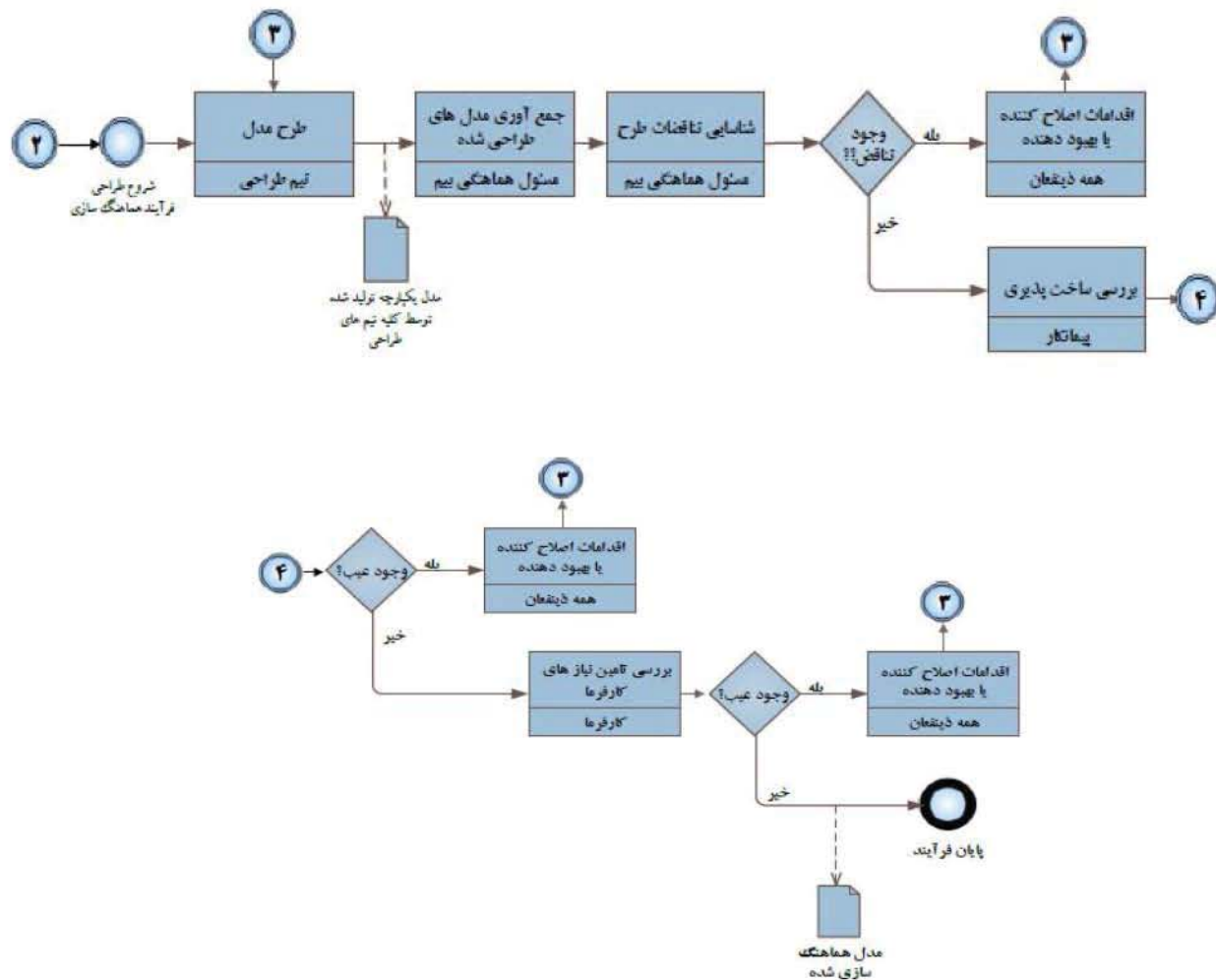
شکل ۳-فلوچارت‌های طراحی بر پایه IDP و BIM
